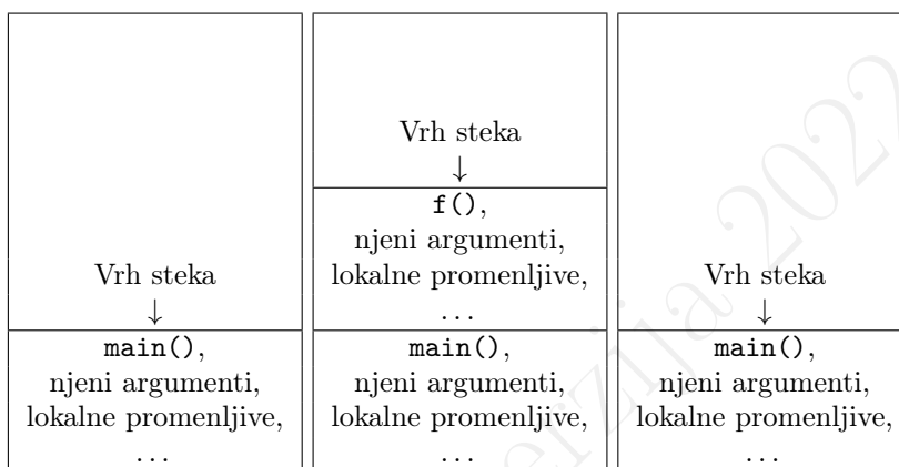
Slika 9.1: Organizacija steka i ilustracija izvršavanja funkcije. Levo: tokom izvršavanja funkcije \text{main}() . Sredina: tokom izvršavanja funkcije f() neposredno pozvane iz funkcije \text{main}() . Desno: nakon povratka iz funkcije f() nazad u funkciju \text{main}() .
